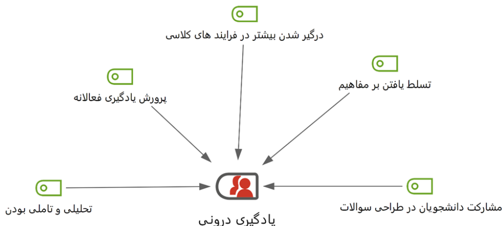
شکل ۴: یادگیری درونی
